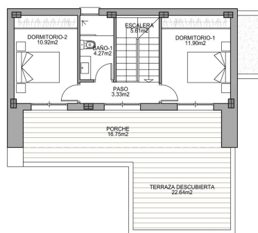
PLANTA PRIMERA
