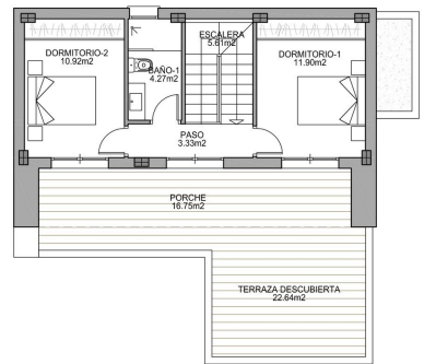
PLANTA PRIMERA
